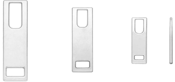
NMR28 DR8 NMR30 DR5 NMR128 DR3
