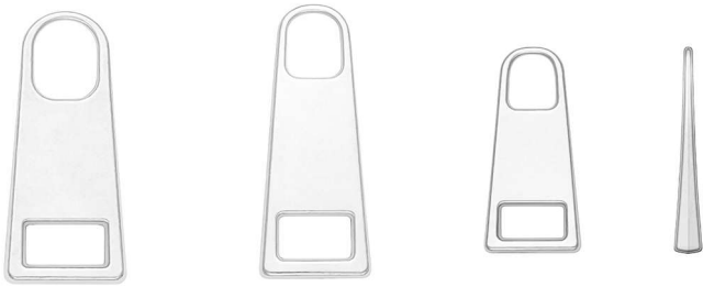
NMR479 DR5-8 NMR227 DR5 NMR229 DR3
